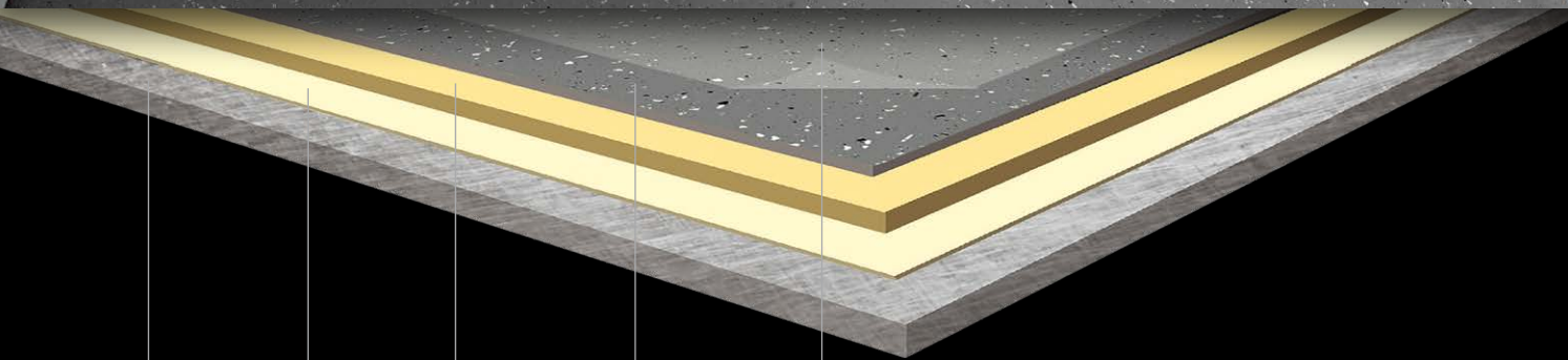
Ondergrond Primer Uitvlaklaag (optioneel) Gietlaag (vlokken optioneel) Topcoat
