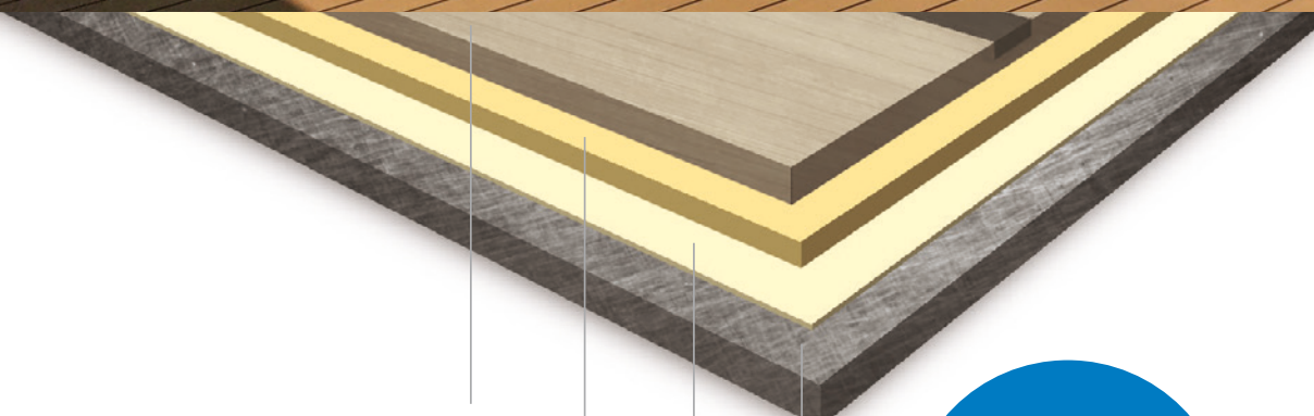
Poured layer Levelling course Primer Foundation
